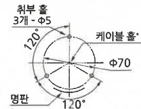
취부면 치수도
