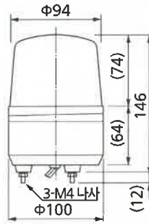
취부면 치수도
