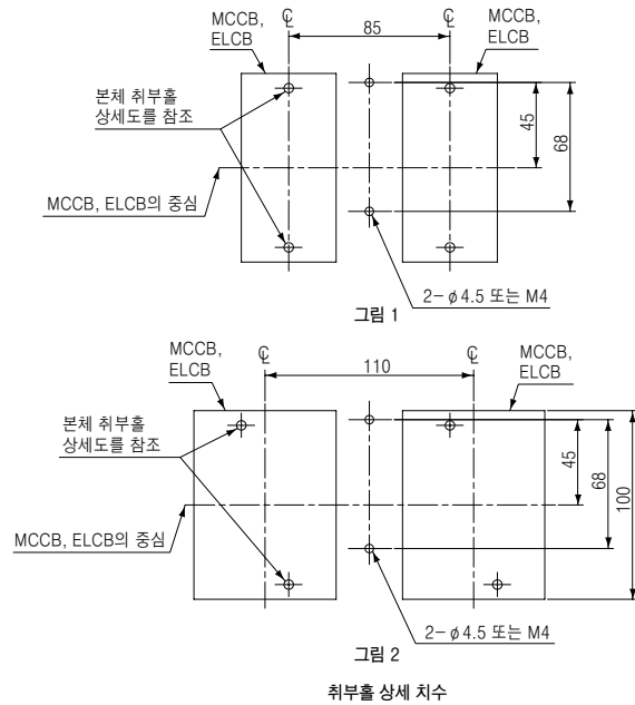
취부홀 상세 치수
