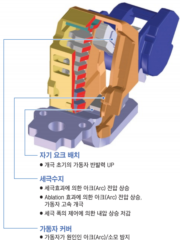
정격전압 480V BW250RAGU (W105×H181×D68mm)
